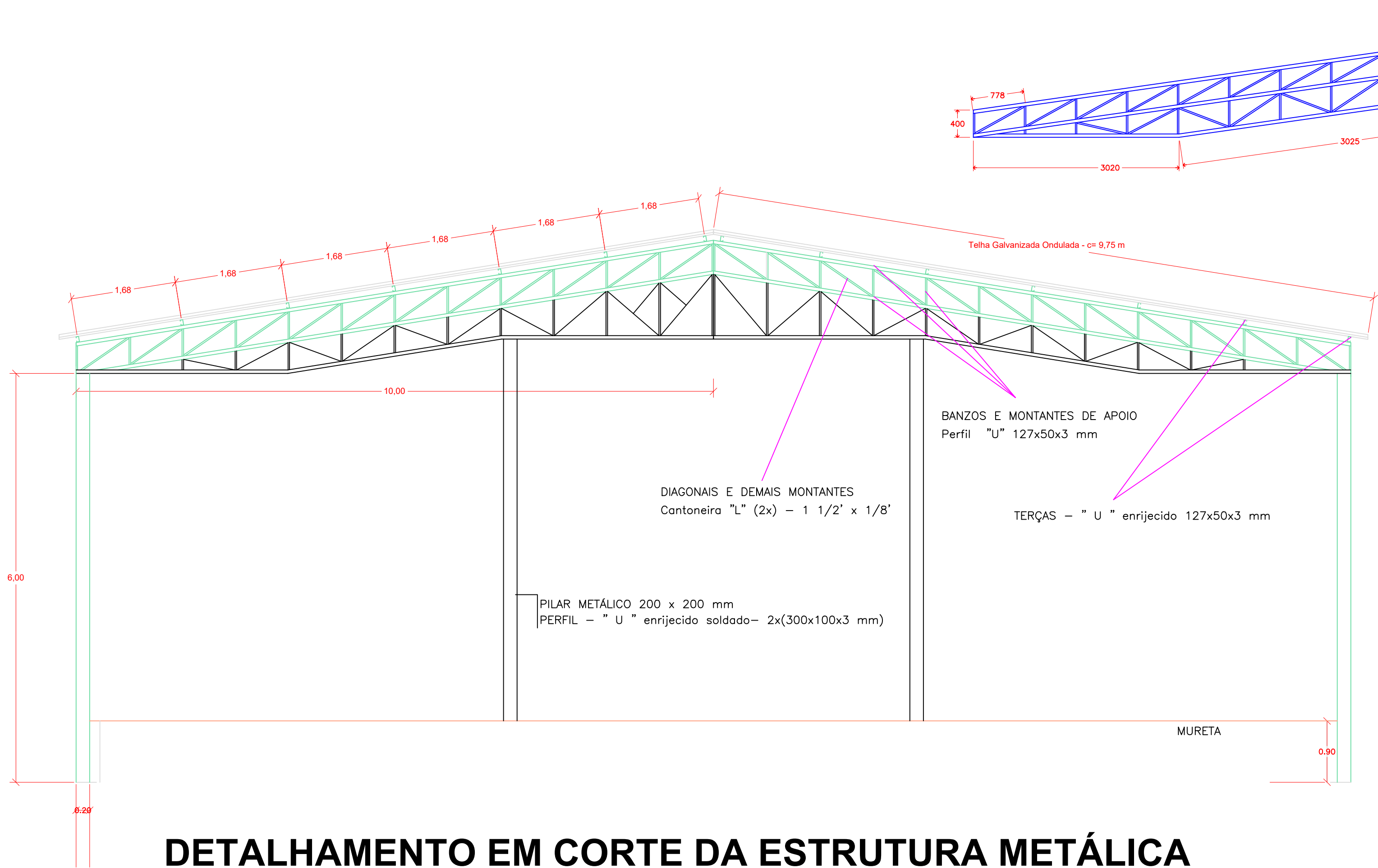
DETALHAMENTO EM CORTE DA ESTRUTURA METÁLICA
