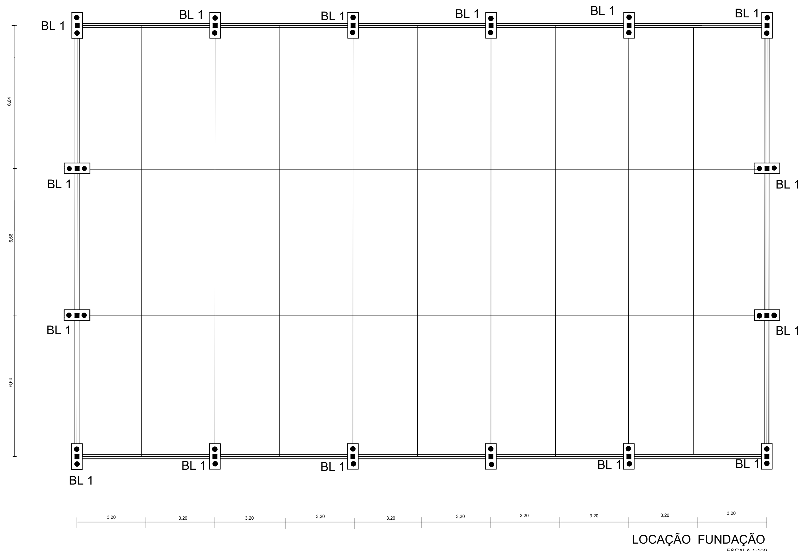
LOCAÇÃO FUNDAÇÃO ESCALA 1:100
